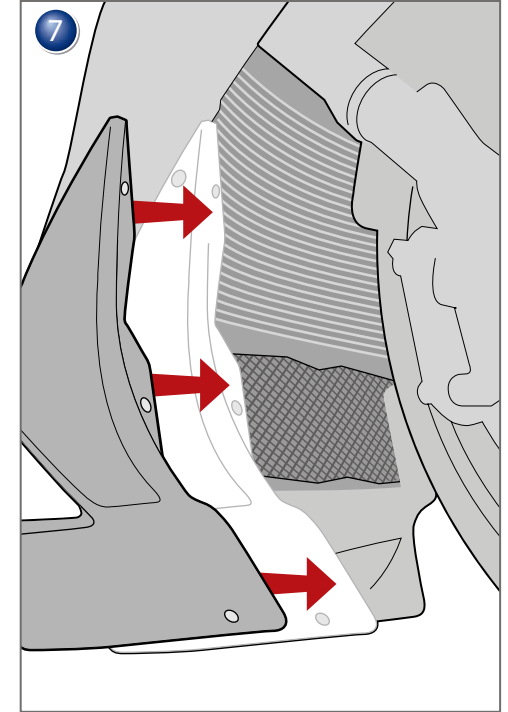
Protección del radiador del aceite Pieza 31961-002
