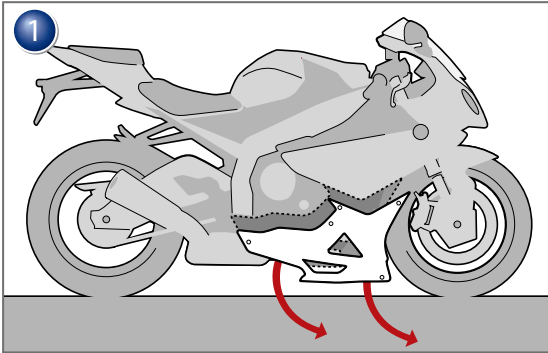
Ölschutzgitter Bestellnummer 31961-002
